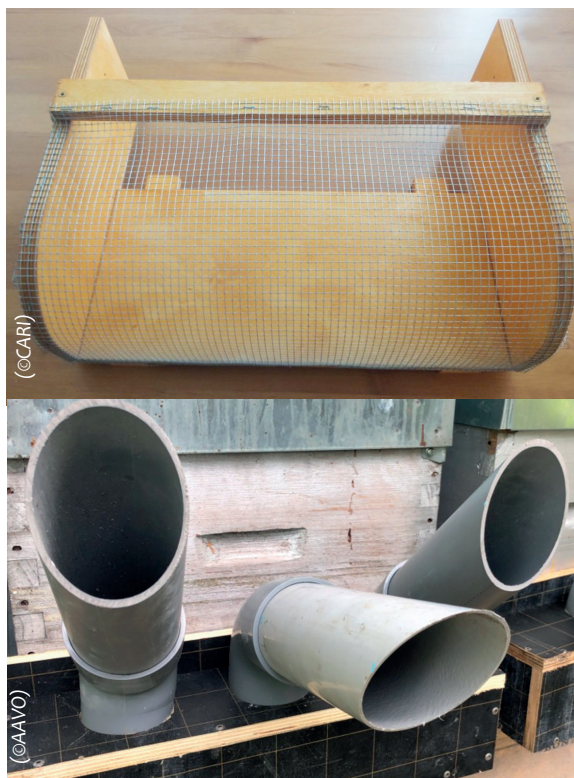
Fig. 2 : Muselières à grillage (haut) et à tube Norma (bas)
